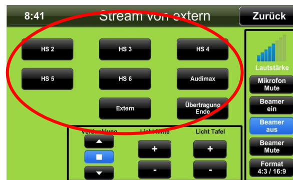
2. Auswahl Hörsaal
